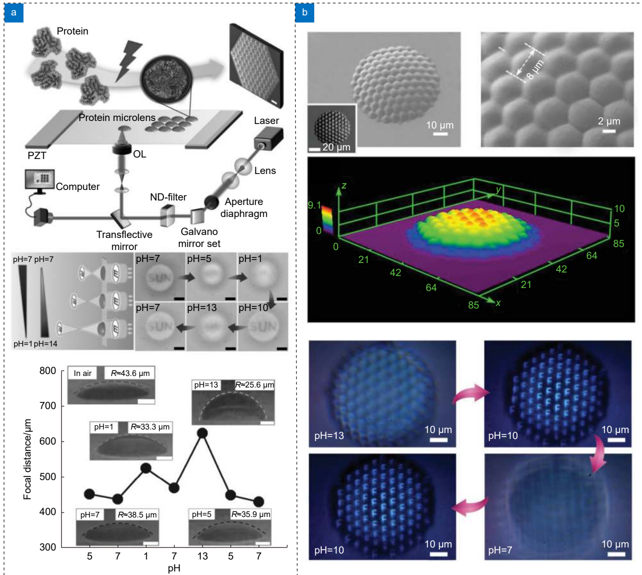
图9 飞秒激光双光子聚合加工微透镜。
