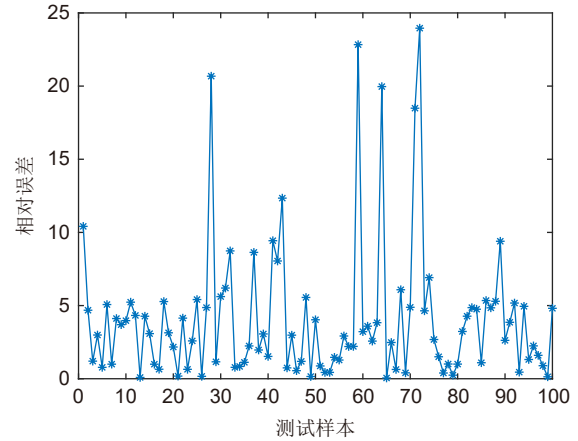
图 5 BP 神经网络预测相对误差 Fig. 5 Relative error of BP neural network prediction
