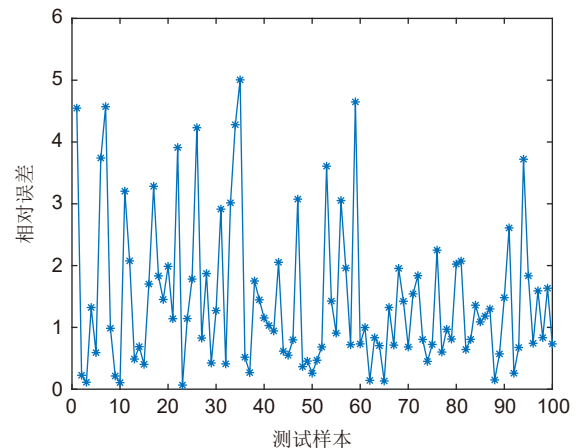
图 7 CS-BP 神经网络预测平均相对误差 Fig. 7 Relative error of CS-BP neural network prediction
