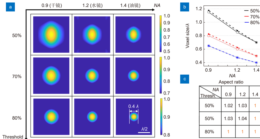
图 3 (a)~(b) x - z 平面上叠加生成的球形焦点的二维光场强度分布, 以及在不同阈值和不同物镜 NAs 下的横向和纵向尺寸大小, 虚线是纵向尺寸、实线是横向尺寸; (c) 在不同的阈值强度和数值孔径下的角向偏振光与径向偏振光焦点的纵向和横向半高全宽的比值
