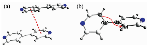
图 5 (a) BP/PFP 共晶中 BP 分子间的作用形式, BP 直接距离(虚线)为 4.3055 \text{ \AA} , 垂直距离为 3.7016 \text{ \AA} ; (b) BP/PFBA 共晶中 BP 分子构象和夹角 C9-C10-C10-C11 扭曲角为 143.769^\circ
