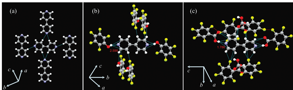
图 4 BP (a), BP/PFP (b) 及 BP/PFBA (c) 的晶体结构图
