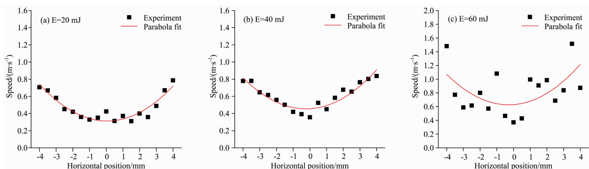
图 6 泵浦能量为 (a) 20 mJ, (b) 40 mJ 和 (c) 60 mJ 时高度为 4 mm 处的火焰水平速度分布
