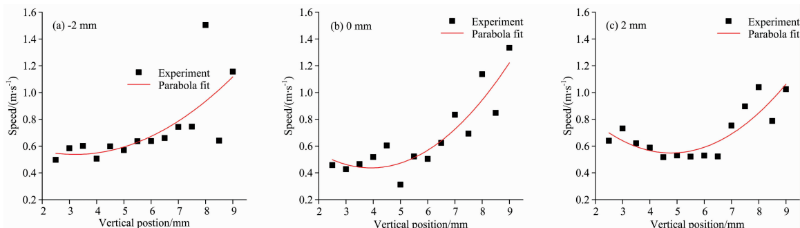
图 5 距离竖直中轴线水平间距 (a) -2 mm, (b) 0 mm 和 (c) 2 mm 处竖直平面的火焰速度随高度分布
