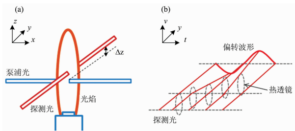
图 1 光热偏转光谱法泵浦探测原理示意图
