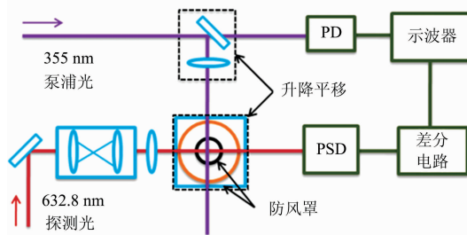
图 2 煤油火焰速度测量实验装置示意图
