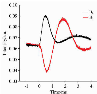
图 3 探测光与泵浦光重合 ( H_0 ) 和位于泵浦光上方 ( H_1 ) 时的时域偏转波形
