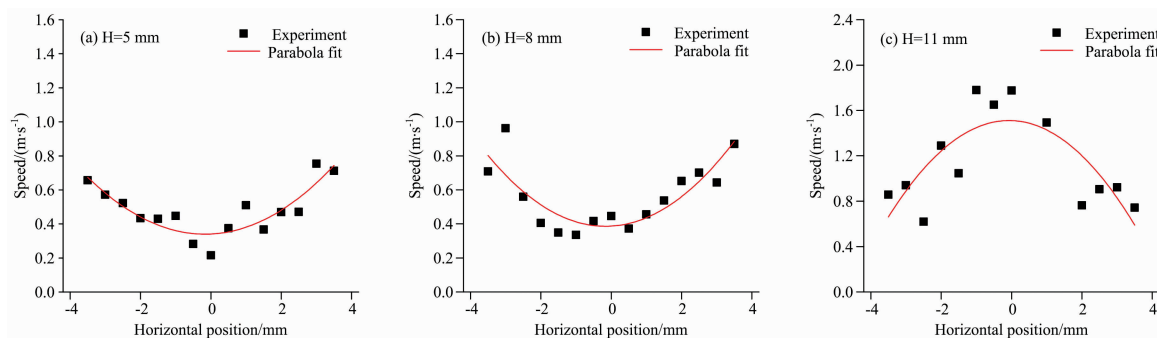
图 4 距离火焰底部高度分别为 (a) 5 mm、(b) 8 mm 和 (c) 11 mm 处的水平面上的火焰速度随位置分布
