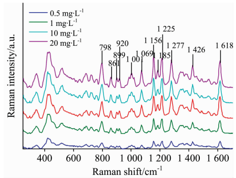
图 3 处理后的专利蓝 V 表面增强拉曼光谱图
