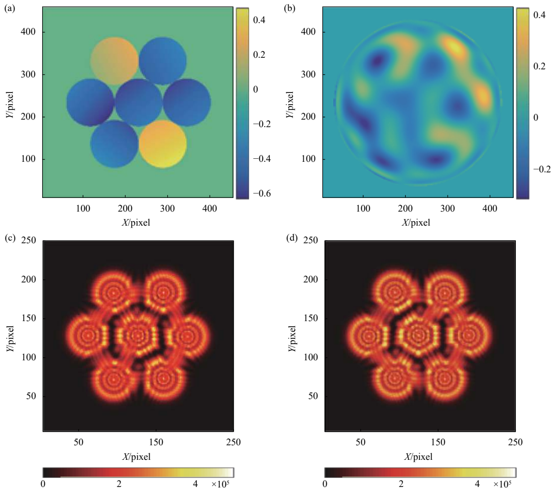
图 5 子镜整体低阶像差感知与调控。(a) 倾斜波前;(b) 重建波前;(c) 焦前光强分布;(d) 焦后光强分布
