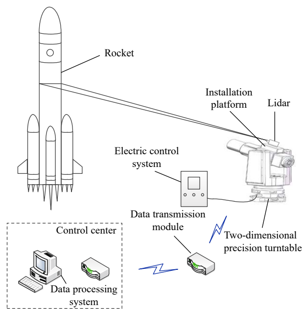
图 2 测量系统组成示意图
