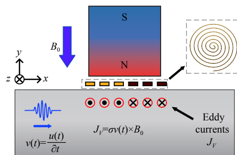
图 2 EMAT 接收换能器工作原理
