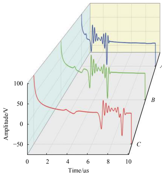
图 13 不同距离节点的电压波形
