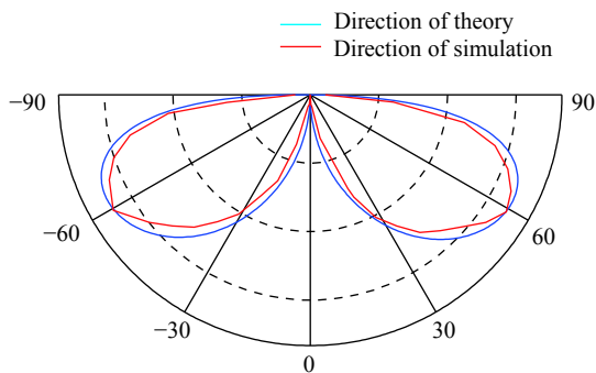
图 8 纵波指向性
