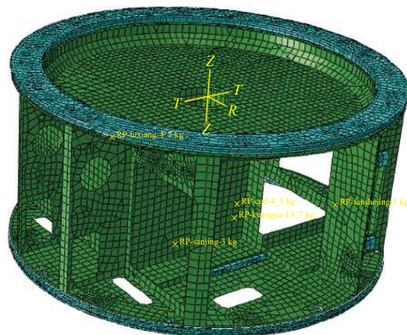
图 7 主支撑结构参数化模型
