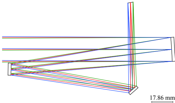
图 14 Buchroeder Schiefspiegler 三镜系统
