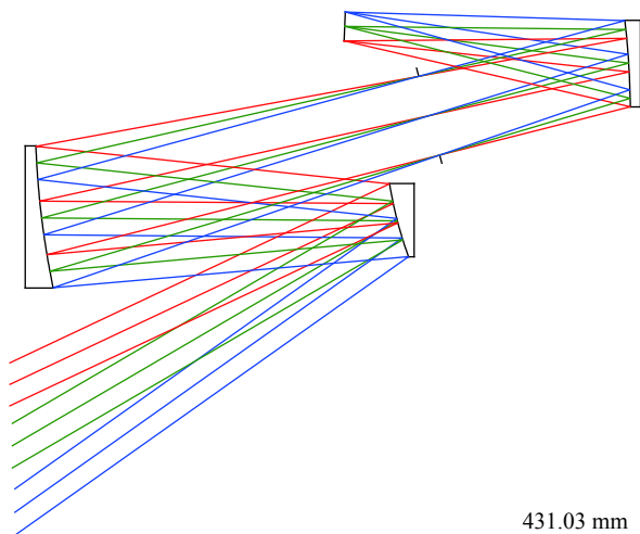
图 23 无中间像面的 Walrus TMA 光学系统 Fig.23 Non-re-imaging Walrus TMA optical system
