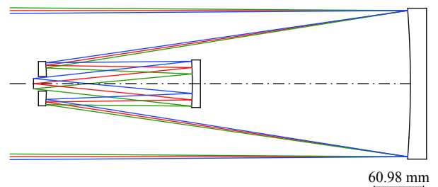
图 5 Korsch 型同轴三镜系统
