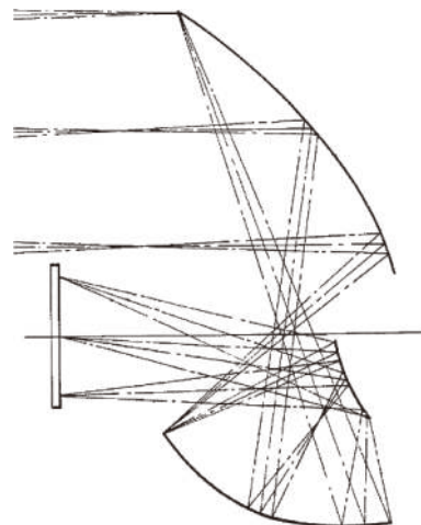
图 28 离轴紧凑型 TMA 光学系统 [32]
