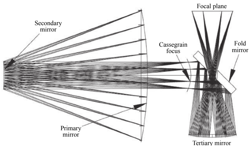
图 11 SNAP 光学系统 [12]
