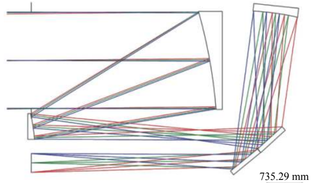
图 36 具有折转镜的离轴 TMA 光学系统 I
