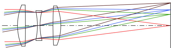
图 18 三片式透镜光学系统
