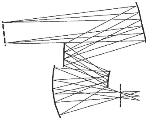
图 35 Cook 于 1996 年提出的离轴 TMA 光学系统 [38-39]
