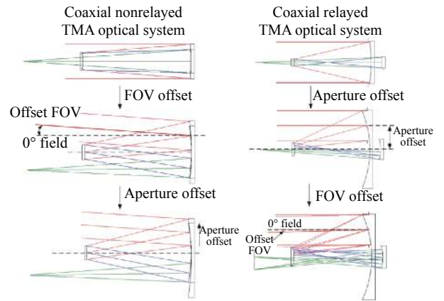
图 16 从同轴系统到离轴系统的转化过程 [15]
