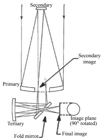
图 10 Korsch 提出的两轴三镜光学系统 II [10]
