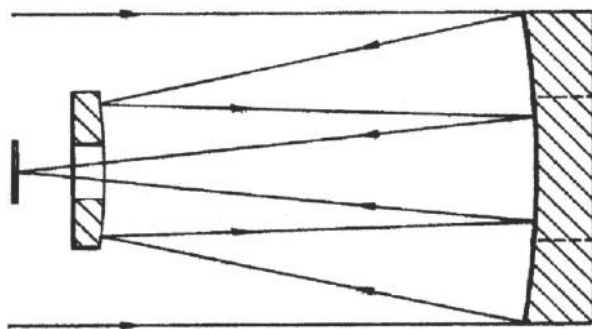
图 4 Rumsey 光学系统 [4]
