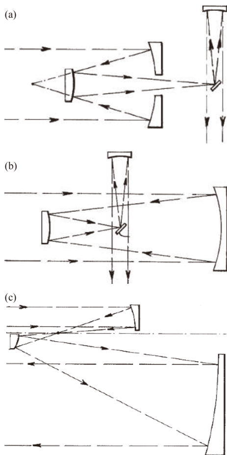
图 38 Abe Offner 提出的 TMA 无焦光学系统: (a) 同轴结构; (b) 同轴结构; (c) 离轴结构 [40]
