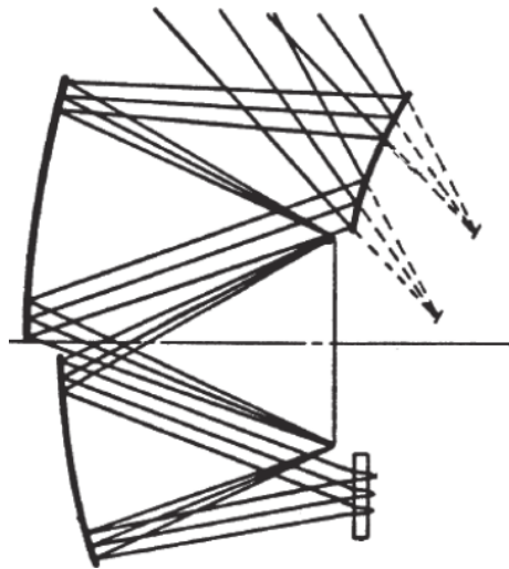
图 34 Cook 于 1994 年提出的离轴 TMA 光学系统 [37]
