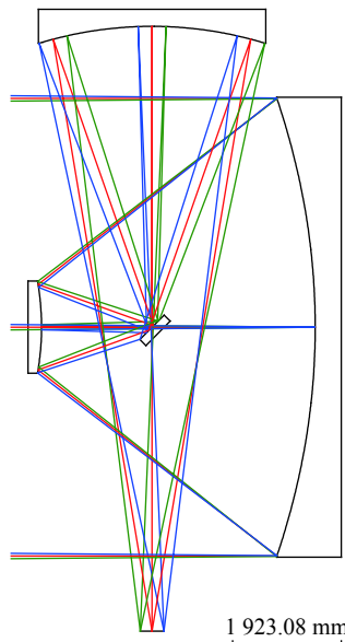
图 7 Korsch 两轴三镜系统
