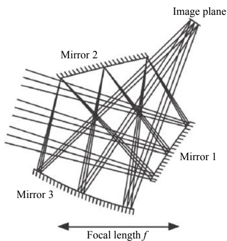
图 31 紧凑型离轴三镜反射式光学系统 [35]
