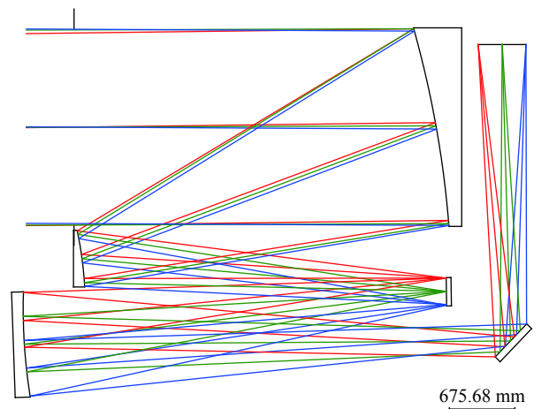
图 37 具有折转镜的离轴 TMA 光学系统 II
