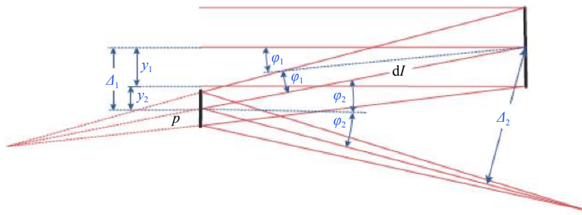
图 13 Schiefspiegler 型光学系统
