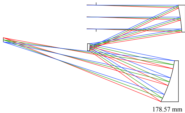
图 27 一次像面在主次镜之间的 TMA 光学系统
