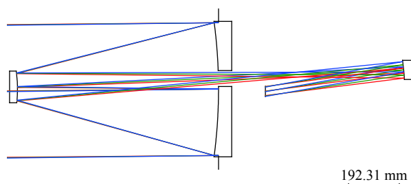
图 39 同轴 TMA 无焦光学系统
