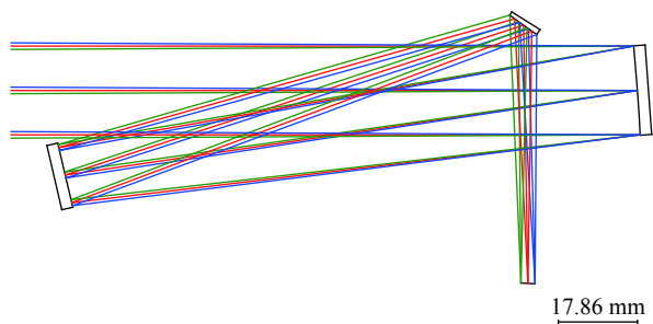
图 15 Solano Schiefspiegler 三镜系统
