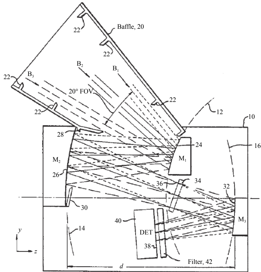
图 22 Hallam 系统 (Hughes Walrus 系统) [22]
