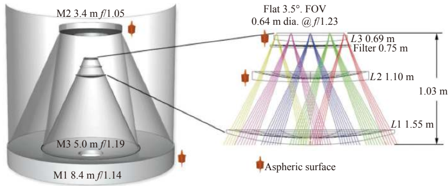
图 3 LSST 光学系统 [3]
