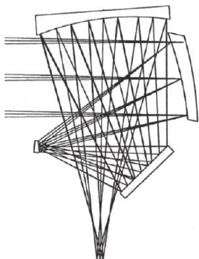
图 30 Rodgers 提出的离轴 TMA 光学系统
