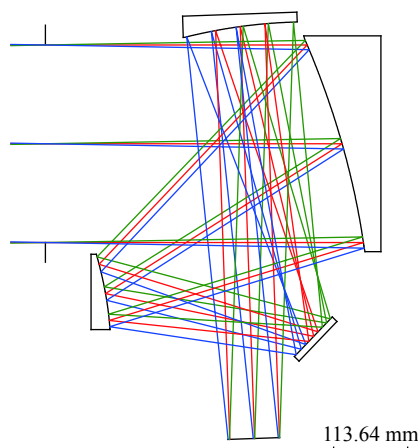
图 40 离轴 TMA 无焦光学系统
