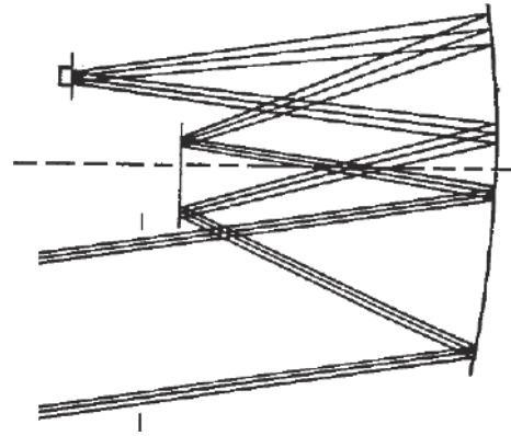
图 21 具有实入瞳的 Cook TMA 光学系统 [21]
