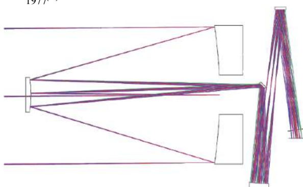
图 9 HiRISE 光学系统
