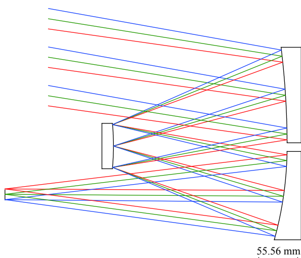
图 19 无中间像面的 Wetherell TMA 光学系统
