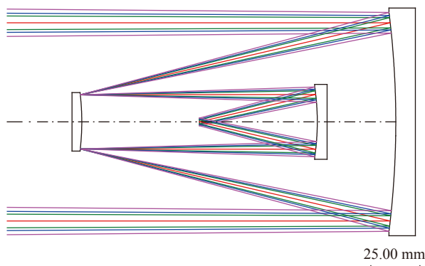
图 1 Paul Baker 三镜系统
