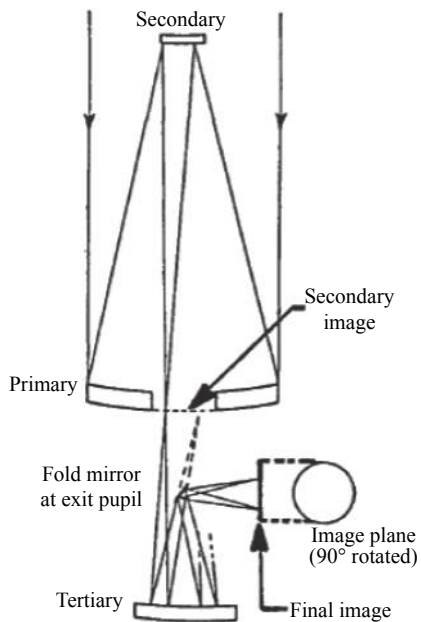
图 8 Korsch 于 1977 年提出的两轴三镜光学系统 I [10]
