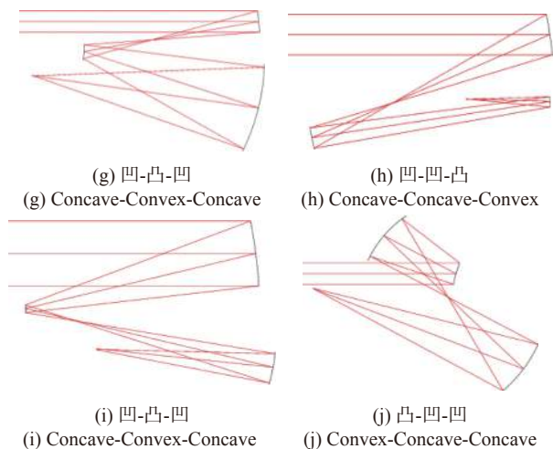
图 17 零匹兹瓦和的离轴 TMA 光学系统结构
