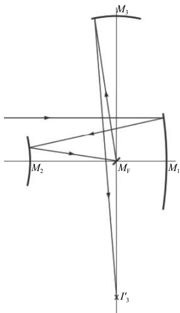
图 6 Korsch 于 1972 年提出的两轴三镜系统 [8]
