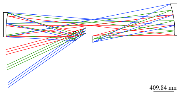
图 29 大视场二次成像离轴 Cook TMA 光学系统
