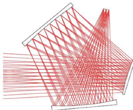
图 32 自由曲面离轴光学系统 [36]
