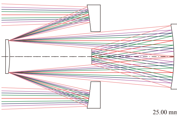
图 2 Willstrop Mersenne-Schmidt 三镜系统
