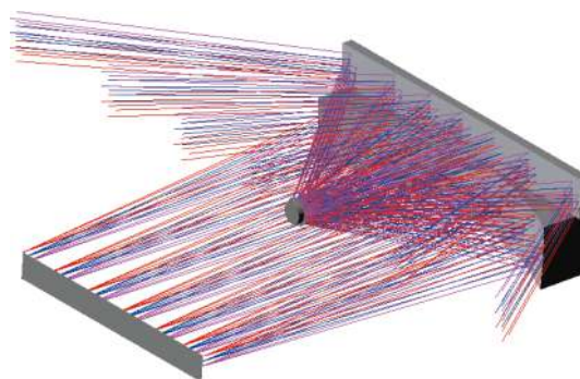
图 20 极大视场离轴 TMA 自由曲面光学系统 [20]
