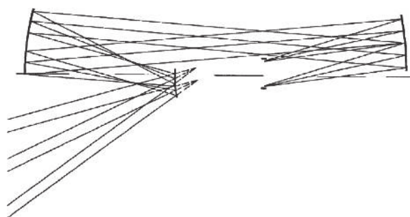
图 41 Cook 提出的离轴 TMA 无焦光学系统 [41]
