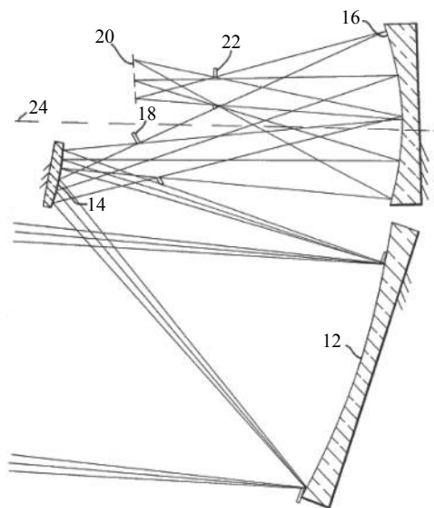
图 25 二次成像的 Cook TMA 光学系统 [25] Fig.25 Re-imaging Cook TMA optical system [25]
