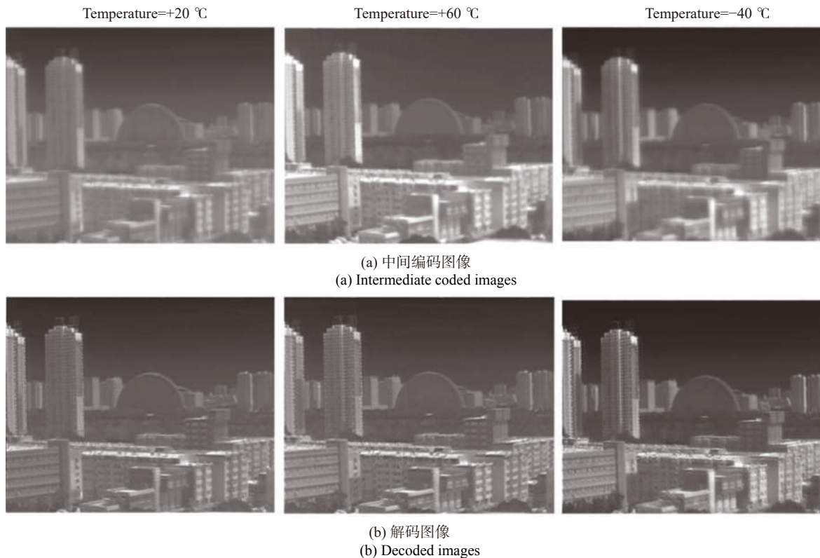
图 13 两透镜大视场波前编码红外成像系统的无热化实验结果 [23]
