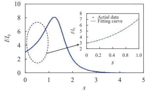
图 3 I/I_0 与 s 关系曲线
