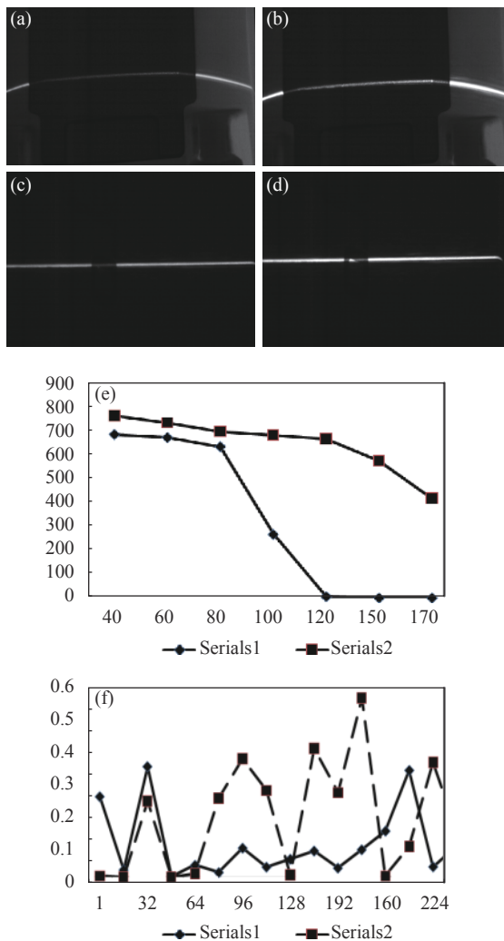
图 8 激光控制器的成像系统成像实验和分析。(a) 异种塑胶材质表面激光投影图像 (21 mA); (b) 异种塑胶材质表面激光投影图像 (55 mA); (c) 包装盒平面激光投影图像 (21 mA); (d) 包装盒平面激光投影图像 (55 mA); (e) 激光光斑有效点数目 (Serials1 表示 (c) 点数, Serials2 表示 (d) 点数) (f) 激光随机测量误差 (Serials1 和 Serials2 分别代表 (c) 和 (d) 误差)
