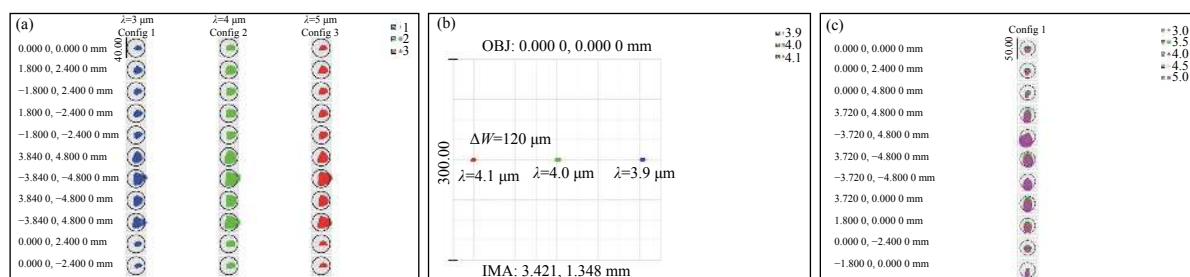
图 6 双光路 Offner 光栅成像系统的点列图
