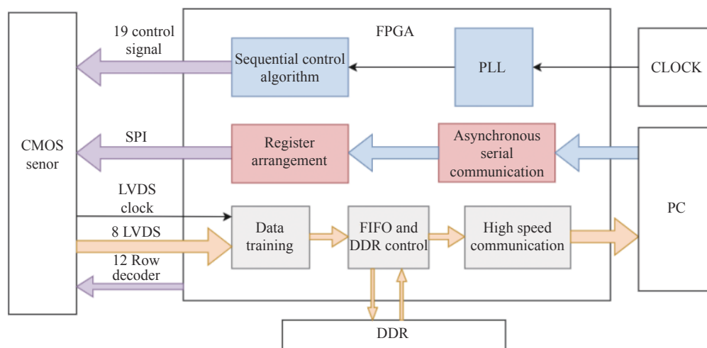
图 3 成像电子学系统功能框图
