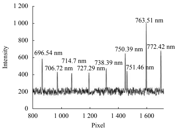
(b) 光谱定标 (b) Spectral calibration
