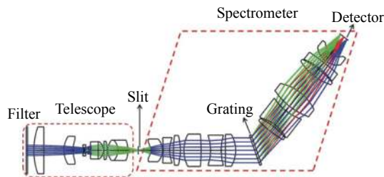
图 4 光学系统图
