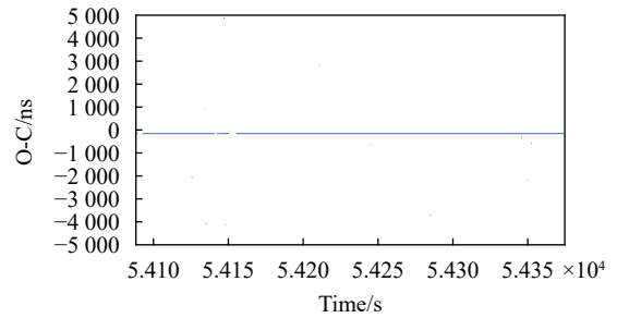
图 3 北斗卫星 compassi6b (~36 000 km) 测距回波信号
