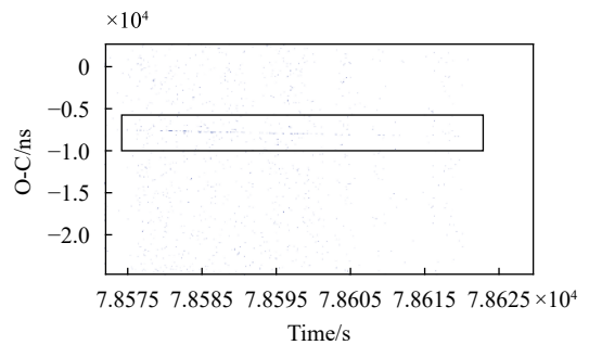
图 4 空间碎片 22 803 (~850 km, 10 m 2 RCS) 的回波信号
