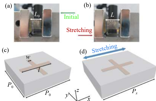
图 2 (a) 样品实物图; (b) 样品拉伸实物图; (c) 可拉伸超表面三维结构示意图; (d) 超表面拉伸变形模型
