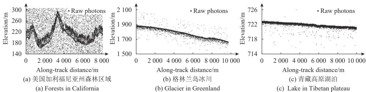
图 2 ICESat-2/ATLAS 数据分布示例
