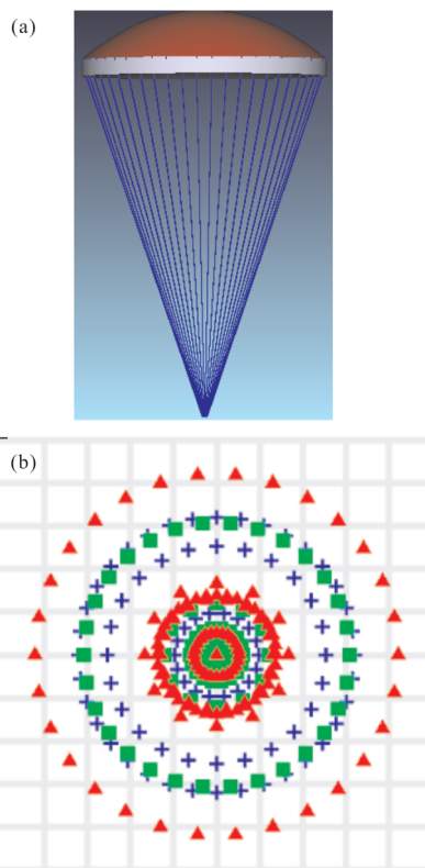
图 4 子眼初始结构光线追迹图及点列图
