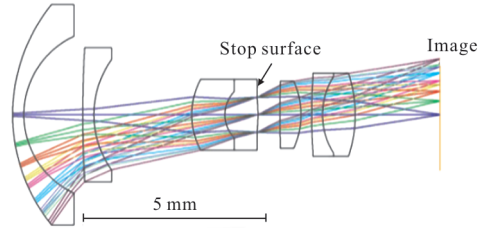
图 8 转像系统光路图
