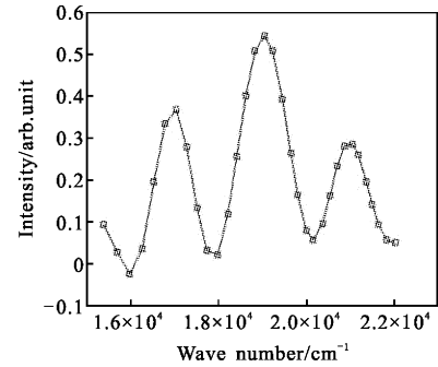
图 5 重构光谱
