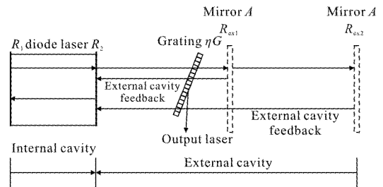
图 3 无输出耦合镜光栅外腔光谱合束结构等效谐振腔
