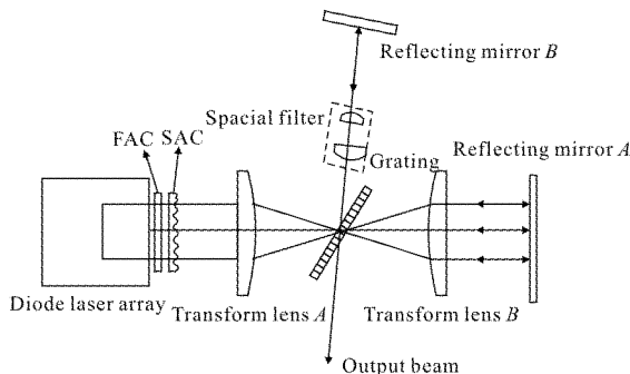
图 2 无输出耦合镜光栅外腔结构光谱合成原理示意图
