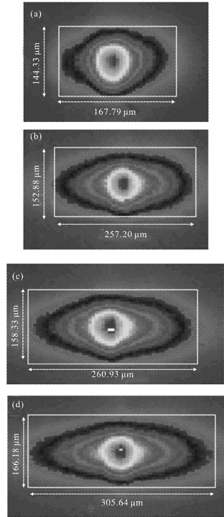
图 7 工作电流分别为 20、30、50、70 A 时合束光束远场光斑 Fig.7 Far field spot of spectral combined beam at pumping current 20,30,50,70 A
