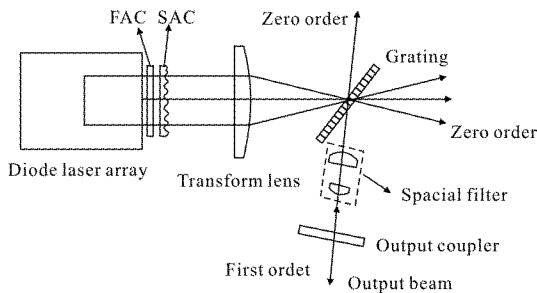
图 1 输出耦合镜光栅外腔结构光谱合束原理示意图
