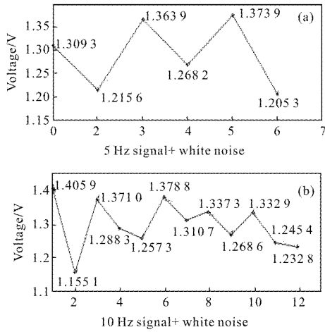
图 4 添加噪声后的直接采样值
