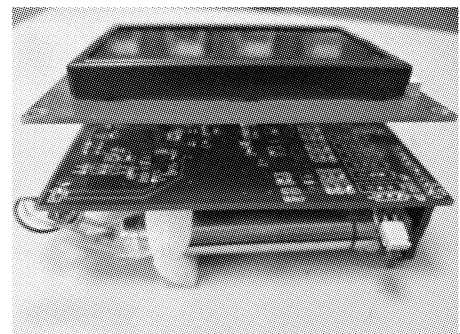
图 6 自制红外热释电气体探测样机
