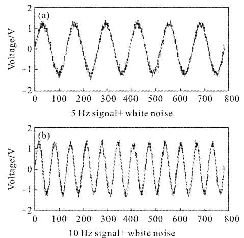
图 3 添加白噪声后的 5 Hz 和 10 Hz 信号
