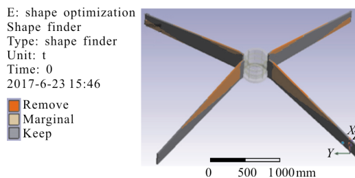
(b) 扭矩载荷
