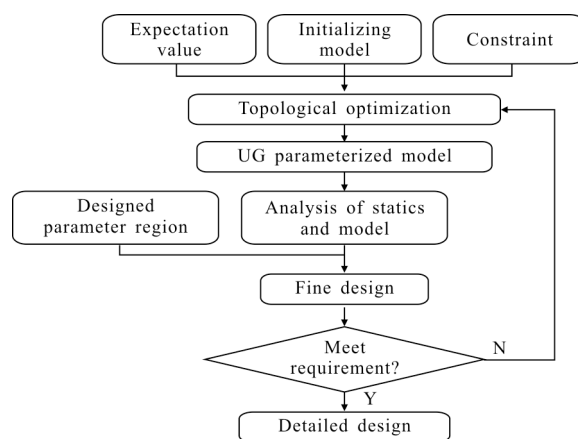
图 4 拓扑优化流程图
