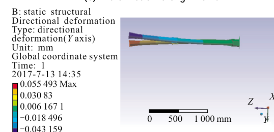
(d) Y 轴向变形 (d) Deformation along Y axis
