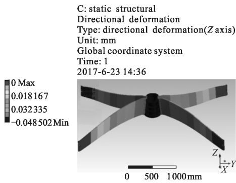
(a) 重力变形
