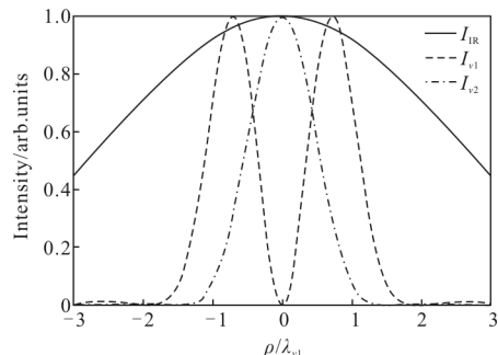
图 4 三束入射光聚焦光场归一化强度分布图
