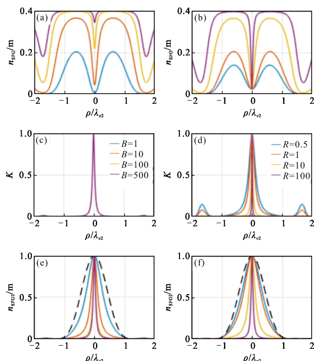
图 6 不同情况下,总和频信号光子流密度 n_{\text{SFG}} , K 值和有效和频信号光子密度 n_{\text{SFG2}} 沿径向 \rho 的变化曲线 Fig.6 Total SFG photon flux density n_{\text{SFG}} , the K value, and useful SFG photon flux density n_{\text{SFG2}} along radial direction \rho at different situations
