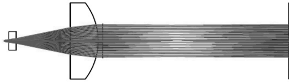
图 5 子午方向光束准直光线追迹
