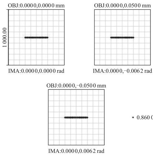
图 6 子午方向光束准直点列图
