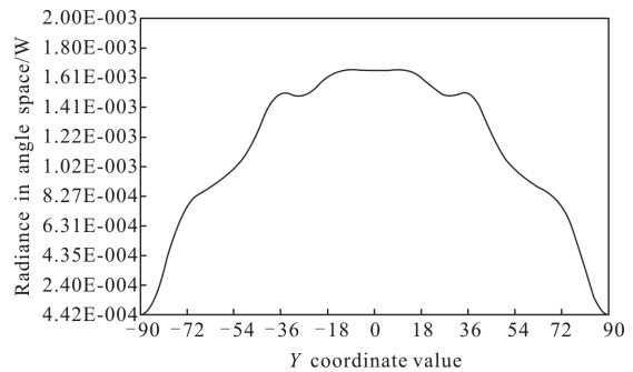
图 8 弧矢方向光束能量分布
