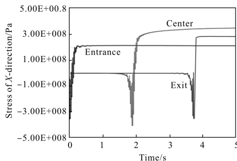
图 5 三个特征点 X 向应力变化曲线
