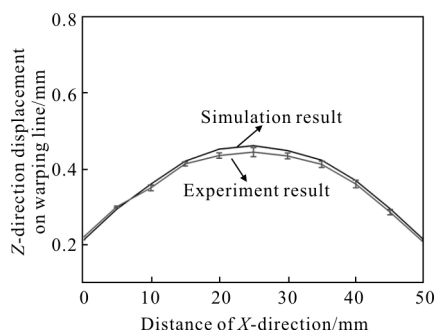
图 8 翘曲线 Z 向位移实验值与模拟值对比
