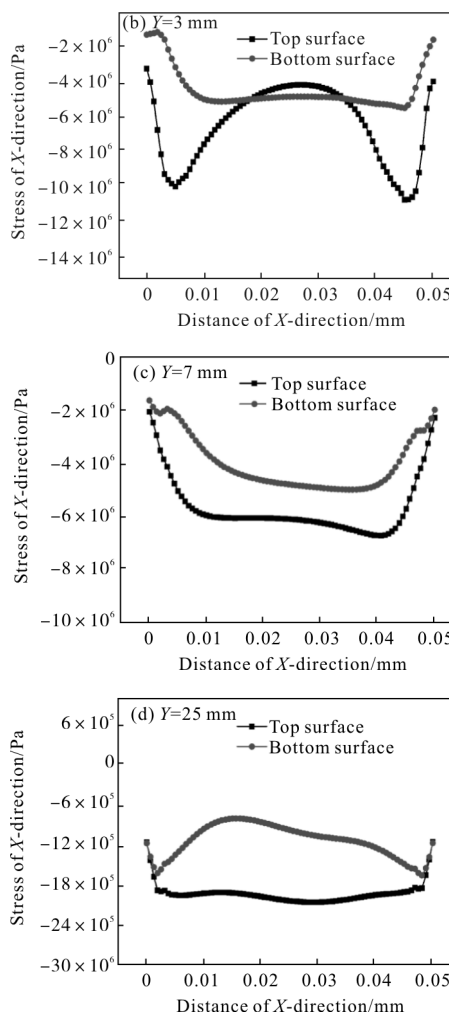
图 6 X 向残余应力
