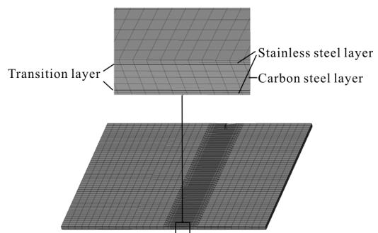
图 1 不锈钢-碳钢复合板的有限元模型
