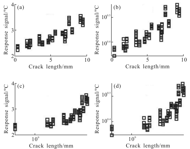
图 4 响应信号随裂纹尺寸的变化
