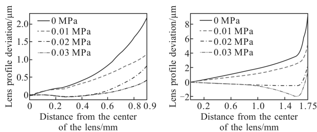
(a) 保持压力对 ASP1 的影响 (b) 保持压力对 ASP2 的影响 (a) Effect of maintenance force on ASP1 (b) Effect of maintenance force on ASP2
