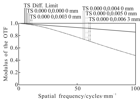
图 5 20 m 距离光学系统 MTF
