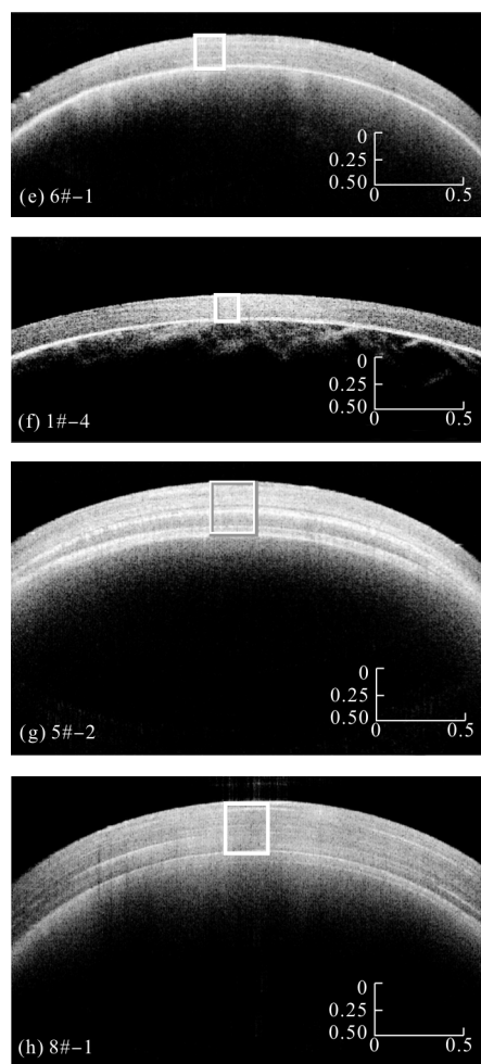
图 6 中国南珠典型 OCT 二维图像
