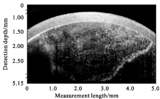
(a) 样品 3#-5 测试区域 1 的 OCT 二维图像 (a) The first test areas OCT 2D images of sample 3#-5
