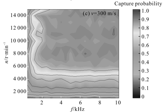
图 10 不同弹速下采用激光周向探测系统时的目标捕获概率
