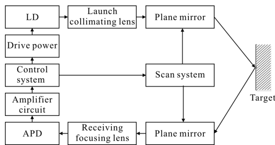
图 2 激光周向探测系统工作原理框图
