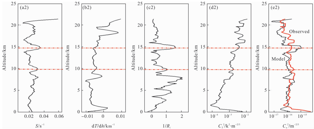
图 1 2016 年 7 月 22 日和 11 月 4 日合肥风切变(a1)、(a2);温度梯度(b1)、(b2); 1/R_i (c1)、(c2);温度结构常数(d1)、(d2)和大气折射率结构常数(e1)、(e2)廓线
