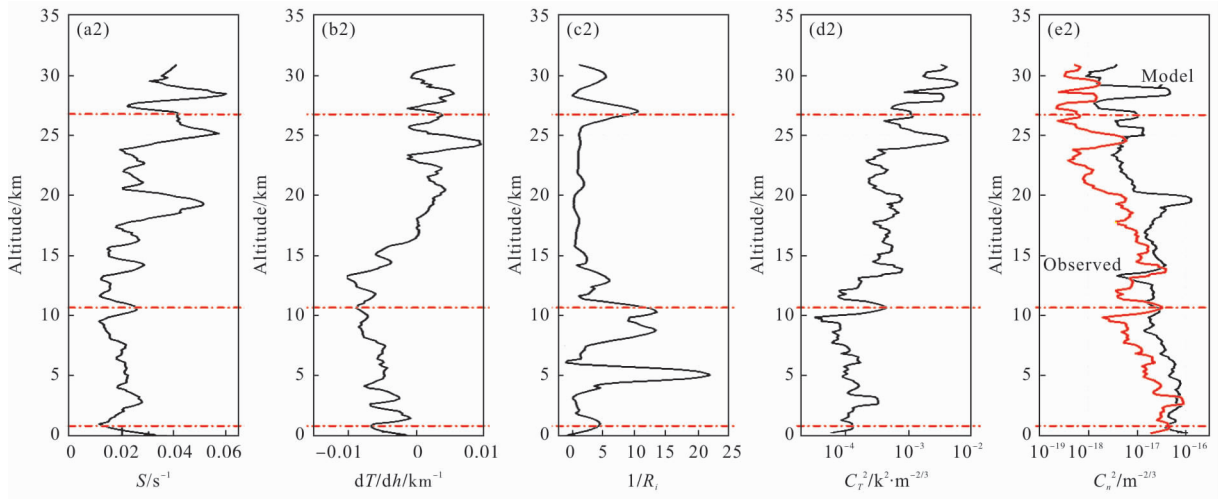
图 2 2016 年 12 月 29 日和 2017 年 1 月 1 日茂名风切变(a1)、(a2); 温度梯度(b1)、(b2); 1/R_i (c1)、(c2);
