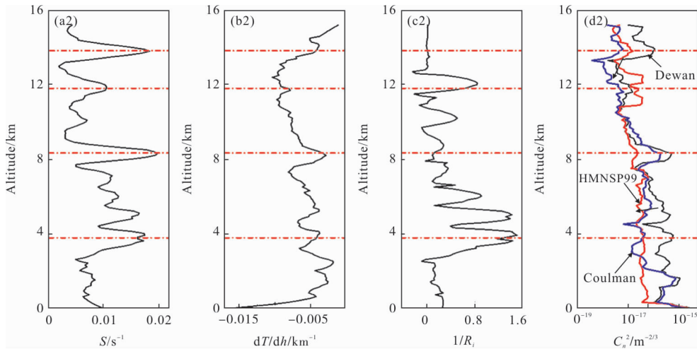
图 4 2014 年 6 月 21 日和 25 日远海海洋风切变(a1)、(a2);温度梯度(b1)、(b2); 1/R_i (c1)、(c2);大气折射率结构常数(d1)、(d2)廓线 Fig.4 Profiles of wind shear (a1),(a2); temperature gradient (b1),(b2); inverse of Richardson number (c1),(c2); refractive index structure parameter (d1),(d2) on June 21 and 25, 2014 on the open sea
