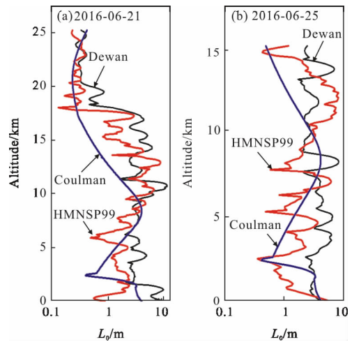
图 3 远海海洋三种外尺度的比较
