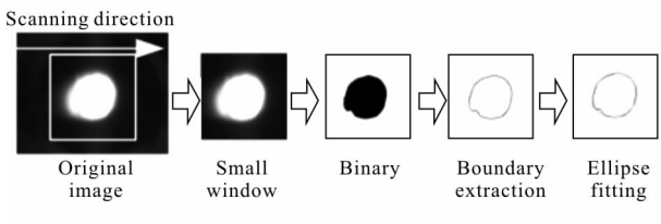
图 2 熔池图像处理过程
