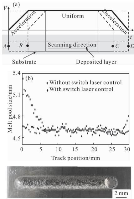
图 4 开关光控制 Fig.4 Switch laser control
