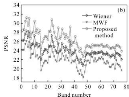
图 7 植被影像采用不同方法滤波后 MSSIM 和 PSNR 值对比
