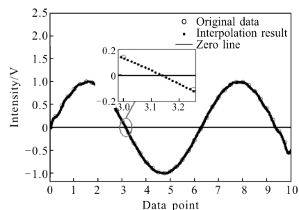
图 2 傅里叶插值
