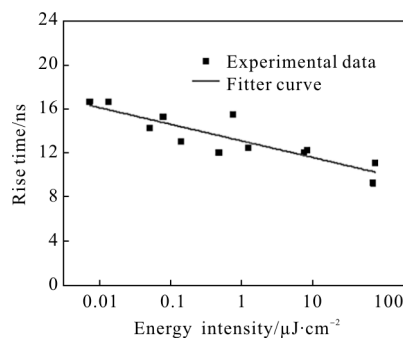
(b) 上升时间 (b) Rise time
