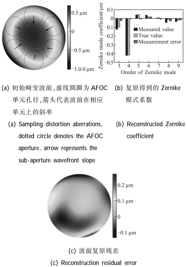
图 12 7 单元 AFOC 阵列波前复原实验结果
