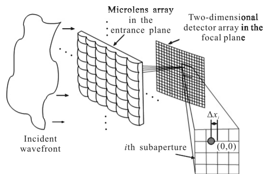
图 10 经典哈特曼传感器的示意图
