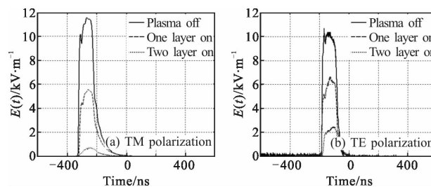
图 4 不同极化条件下透射波形图
