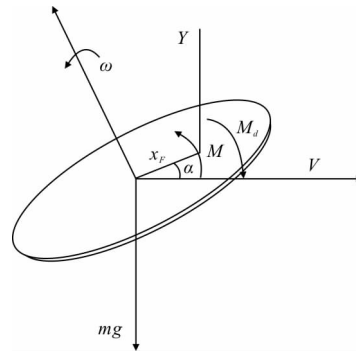
图 3 箔片受力示意图
