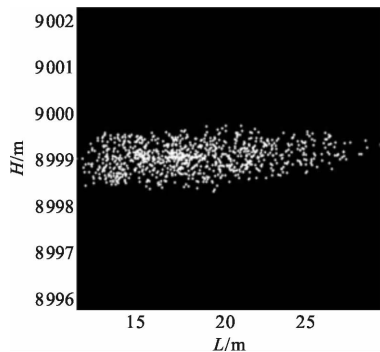
图 12 75°侧向灰度图 Fig.12 75° lateral gray image
