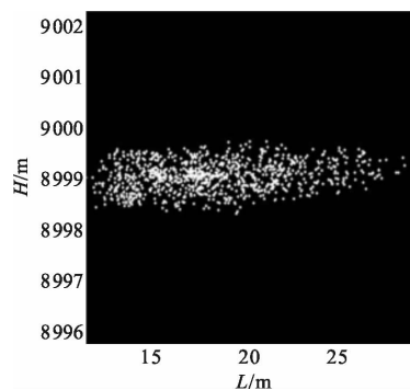
图 13 75°尾后灰度图 Fig.13 75° caudal gray image
