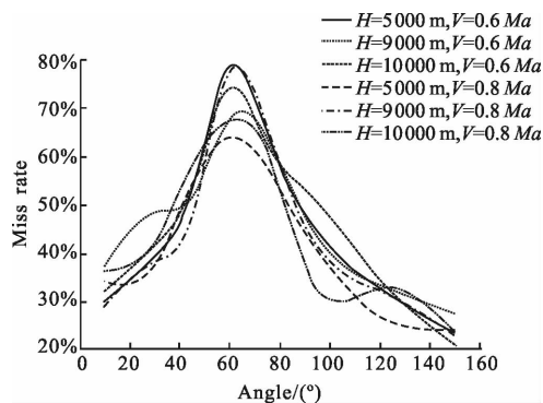
图 14 面源诱饵角度特性曲线
