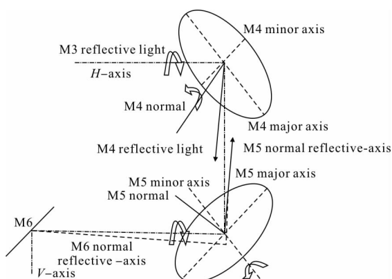
图 3 未对准反射光路
