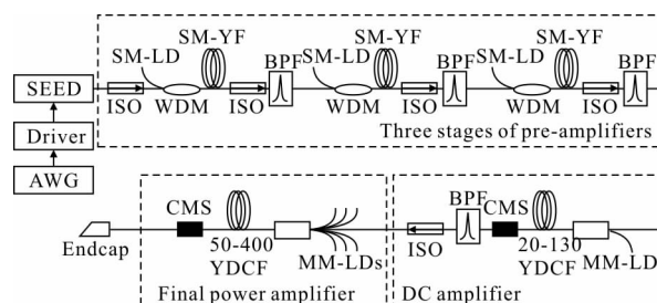
图 9 高功率纳秒短脉冲光纤激光器结构图
