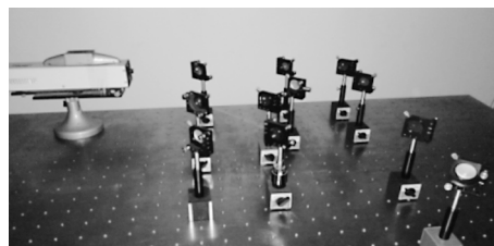
图 6 准平行光干涉实验装置实物图
