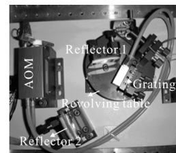
(b) 波长调谐机构实物图
