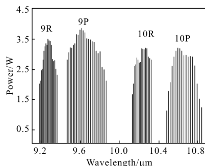
图 5 调 Q \text{CO}_2 激光器输出谱线:光栅设计波长 9.60 \mu\text{m}
