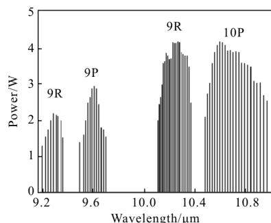
图 4 调 Q \text{CO}_2 激光器输出谱线:光栅设计波长 10.59 \mu\text{m}
