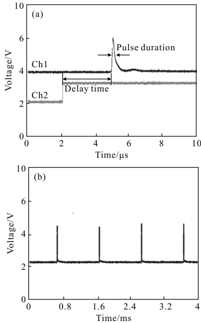
图 6 重频为 1 kHz 时的激光脉冲波形 Fig.6 Waveforms of laser pulses at 1 kHz
