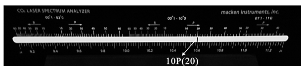
图 3 10P(20)支 \text{CO}_2 激光谱线照相图
