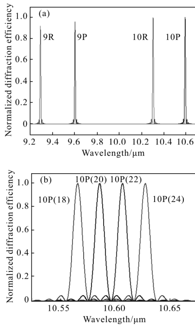
图 1 各谱线激光衍射效率分别随波长变化关系
