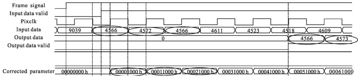
图 5 校正模型模块输入输出波形图
