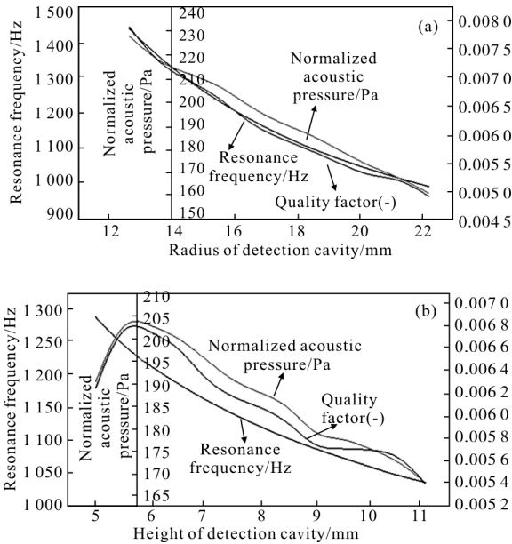
图 6 探测腔结构参数优化
