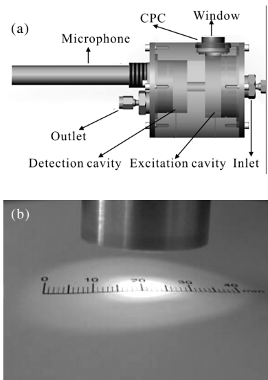
图 2 亥姆霍兹光声池结构设计
