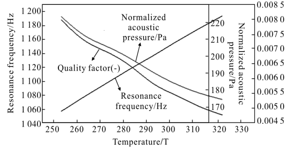
图 7 光声池温度特性
