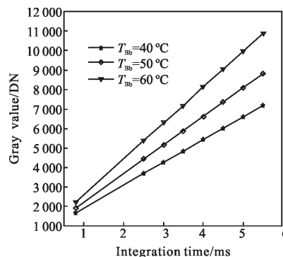
图 5 辐射亮度与输出灰度的关系
