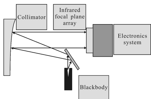
图 1 平行光管法定标
