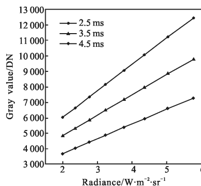
图 4 积分时间与灰度值的关系
