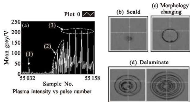
图 3 损伤形态转化过程信号探测
