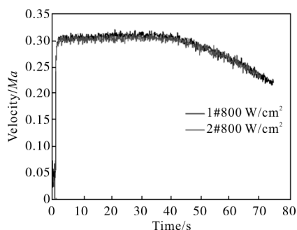
图 6 两次 800 W/cm 2 激光辐照过程中切向气流速度变化
