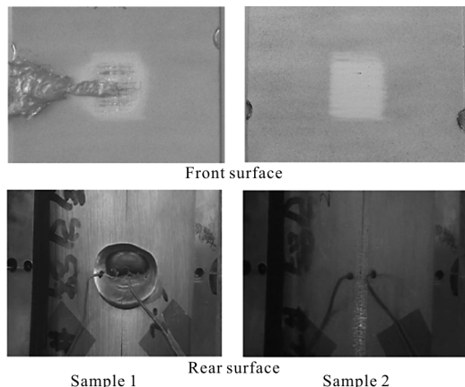
图 3 激光辐照后样品前后表面照片
