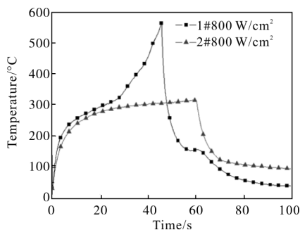
图 7 800 W/cm 2 激光辐照下后表面热电偶测温曲线
