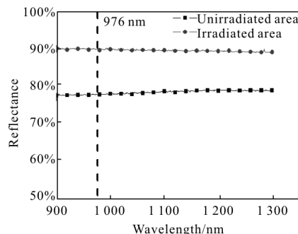
图 8 辐照区与未辐照区涂层的表面反射率谱
