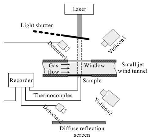
图 1 实验系统示意图
