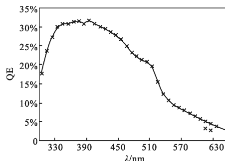
图 4 在双碱阴极的基础上改进的高量子效率光阴极的光谱响应曲线
